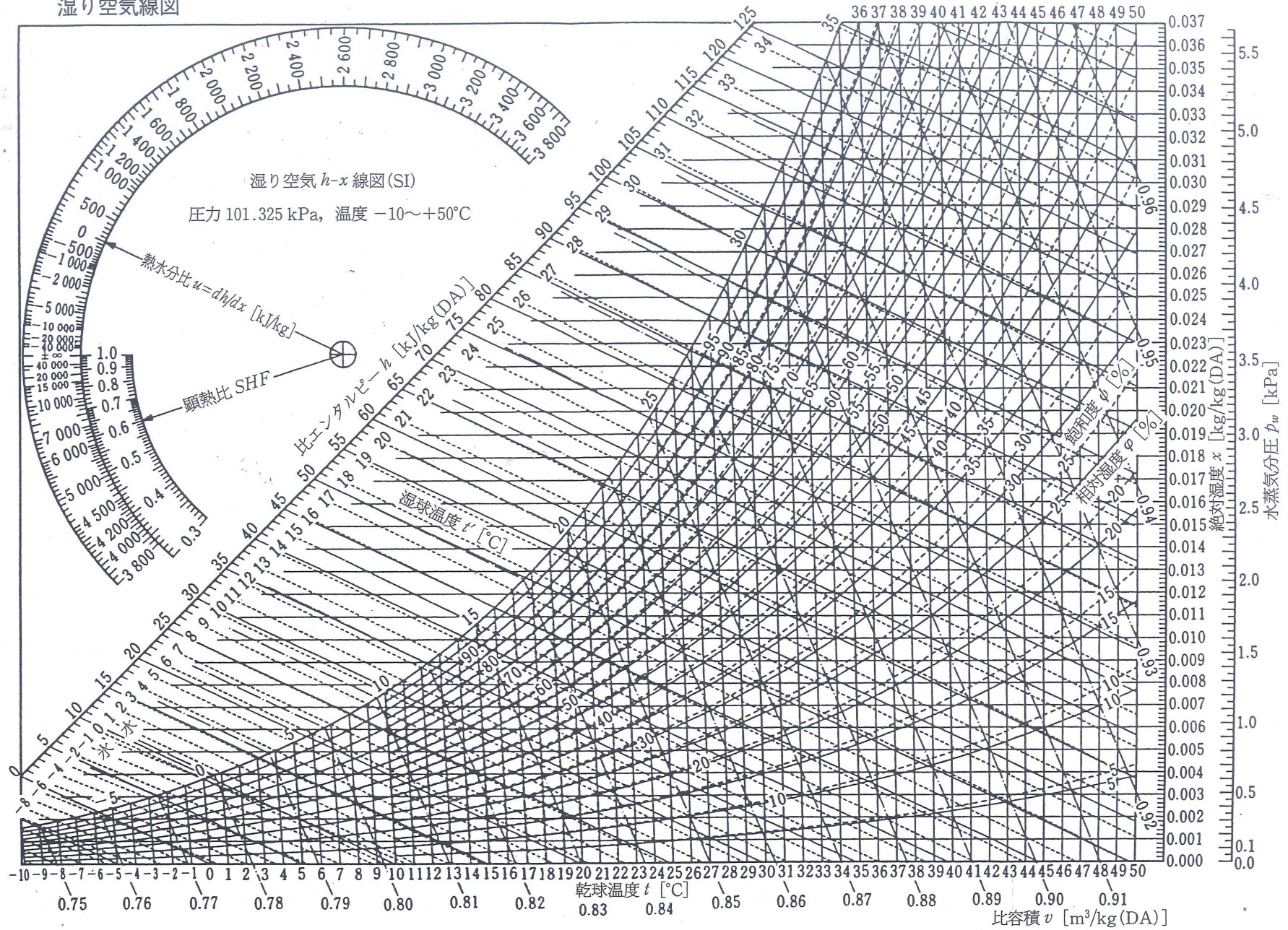
湿り空気線図
